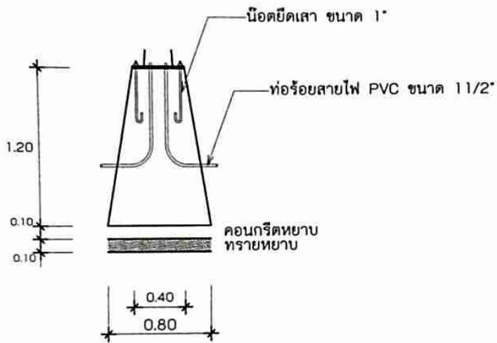
รูปตัดฐานเสาคอนกรีต
