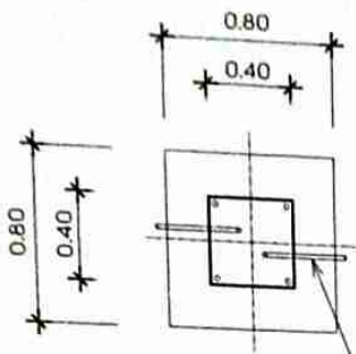
แปลนฐานเสาคอนกรีต
