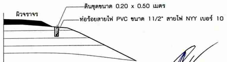
รูปตัดขุดดินเดิมท่อร้อยสายไฟ
